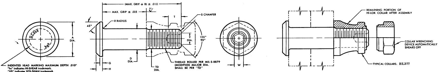
HI-LOK PIN
