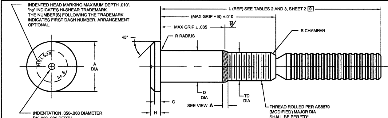
HI-LITE®ST™ PIN
